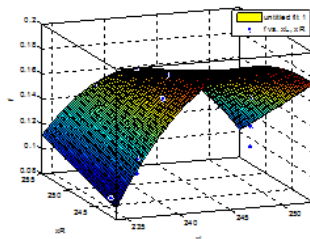
Фиг. 2. Нелинелен модел на отразен сигнал с дължина \lambda = 630 \text{ nm} и сондиращ сигнал с \lambda = 530 \text{ nm}
