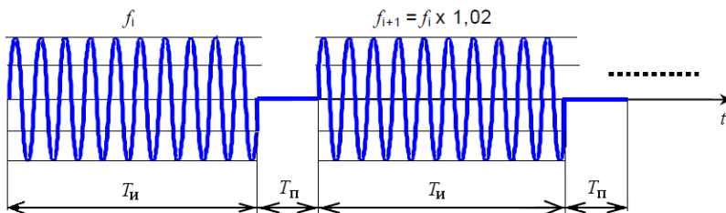
Фиг. 2. Изпитвателна вълна със CW импулси с паузи.
