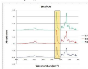
Fig. 1. EtAc/AAc spectrograms
